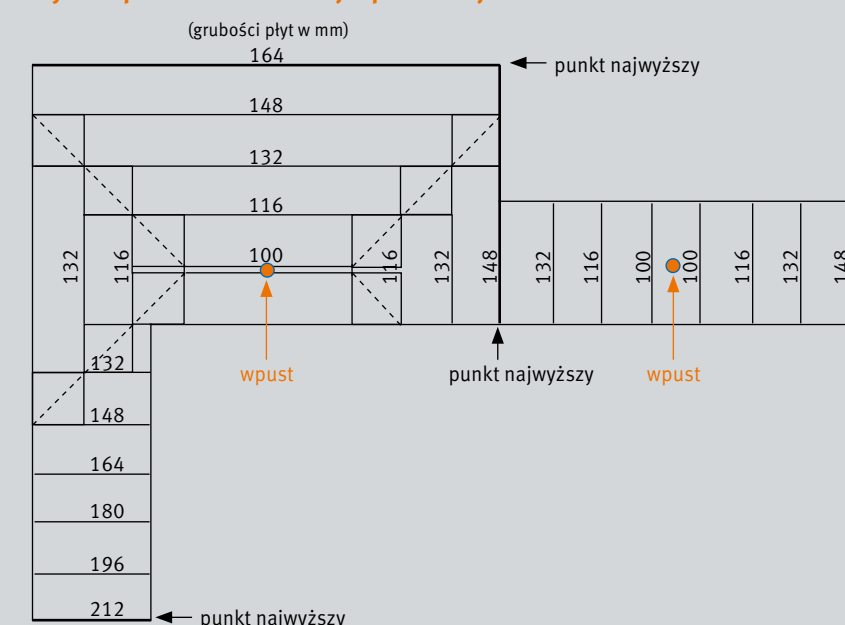
Przykład planu termoizolacji spadkowej:
