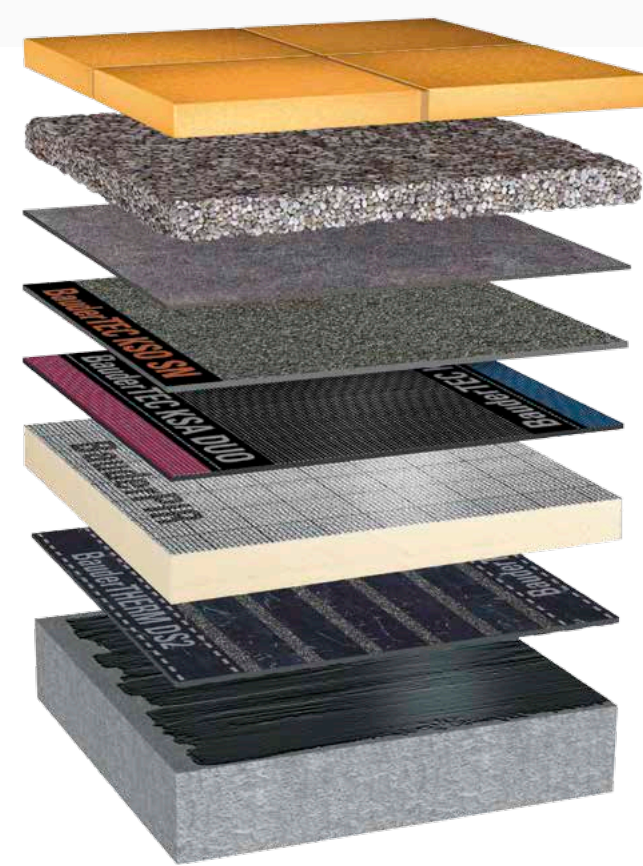
Przykład systemowego układu warstw: BauderPIR FA TE
