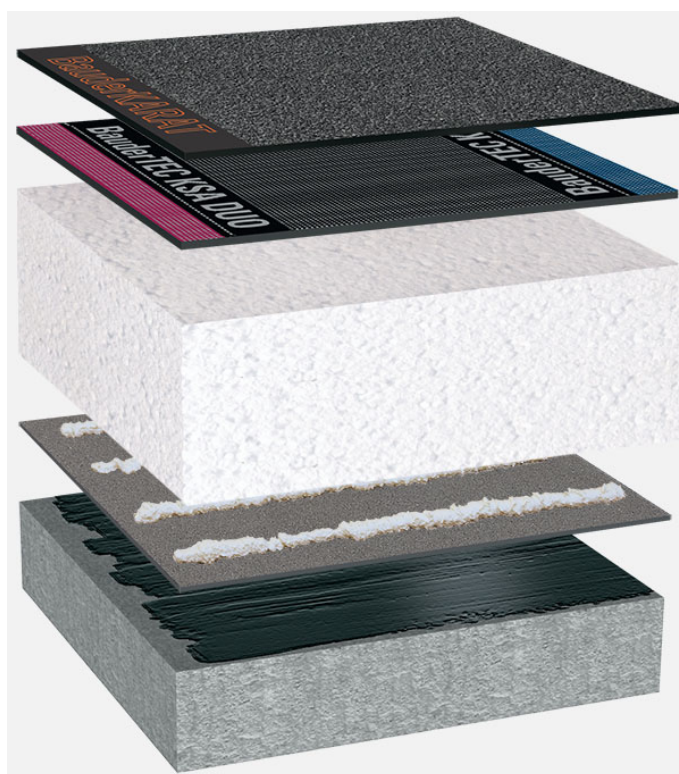
Systemowy układ warstw: BG_EPS-P_K_01
