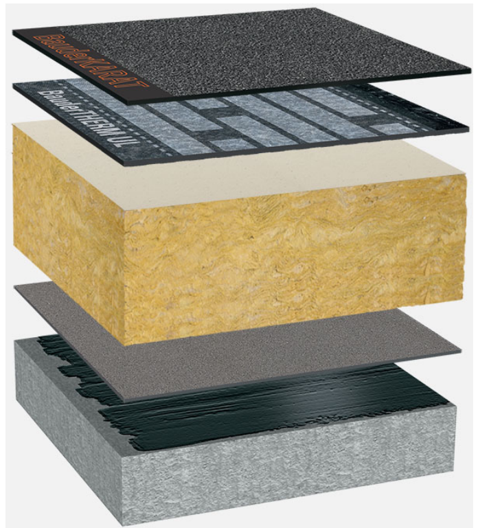
Systemowy układ warstw: BG_MIFA-P_K_01
