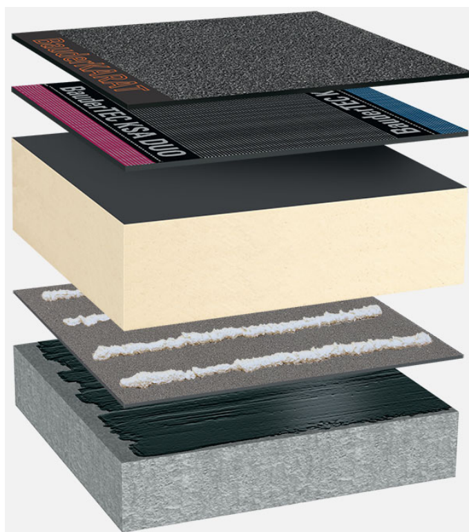
Systemowy układ warstw: BG_PIR-FA_K_01
