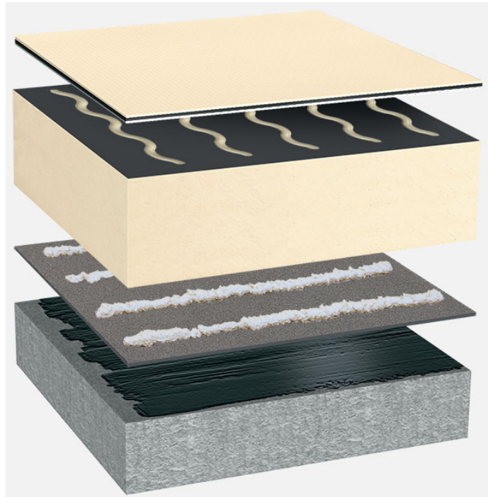
Systemowy układ warstw: BG_PIR-FA_TV_01
