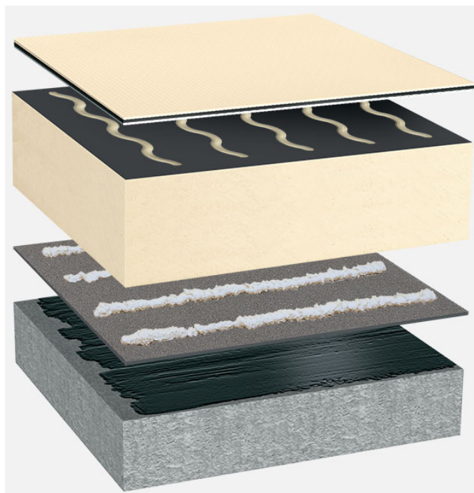
Systemowy układ warstw: BG_PIR-FA_TV_01
