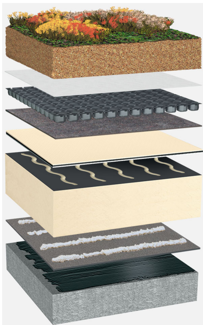
Systemowy układ warstw: BG_PIR-FA_TV_01_G125
