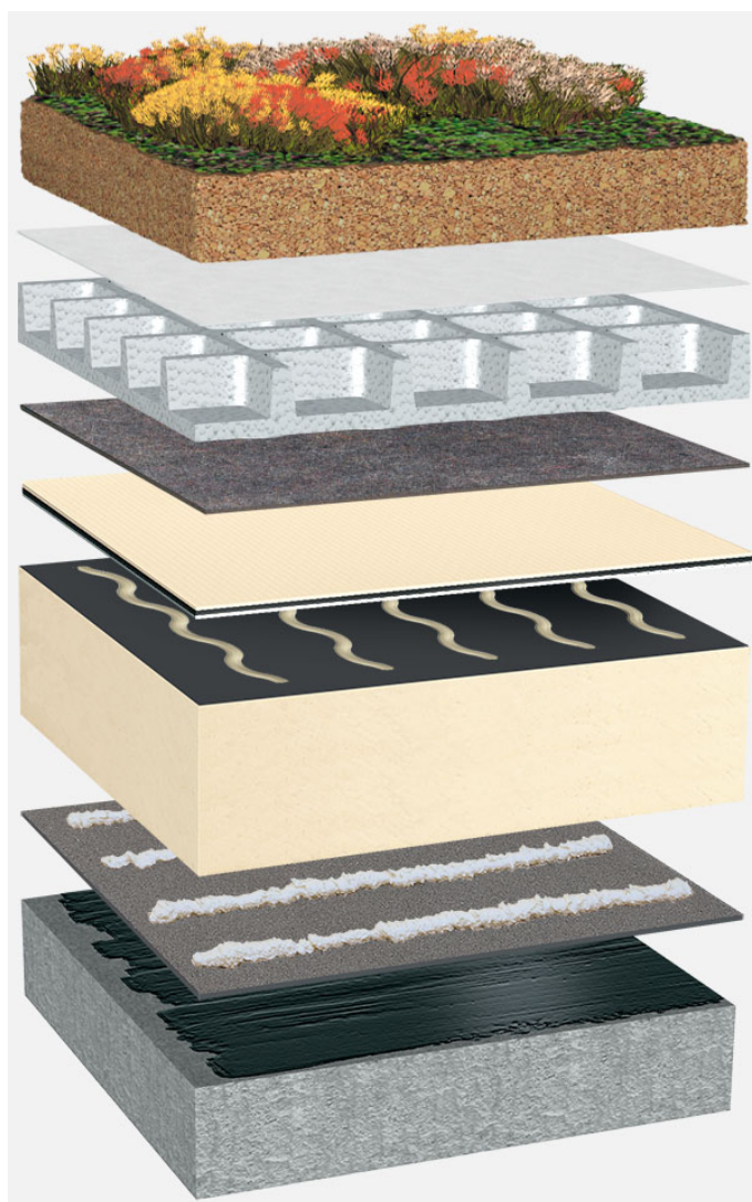
Systemowy układ warstw: BG_PIR-FA_TV_01_G75
