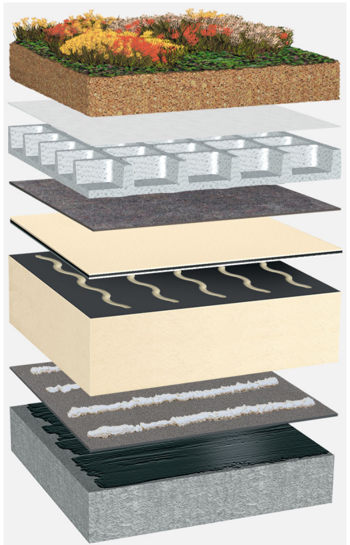
Systemowy układ warstw: BG_PIR-FA_TV_01_G75
