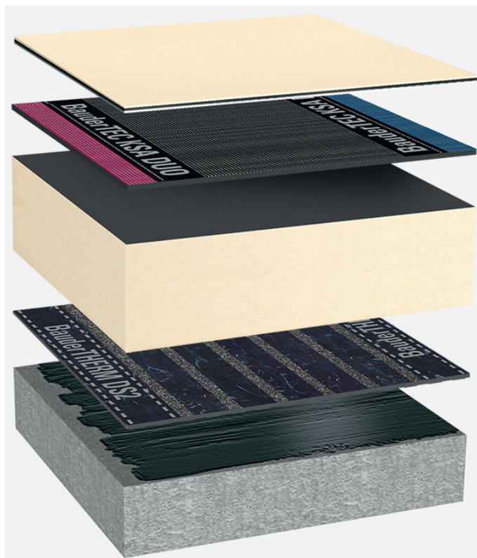
Systemowy układ warstw: BG_PIR-FA_TV_02
