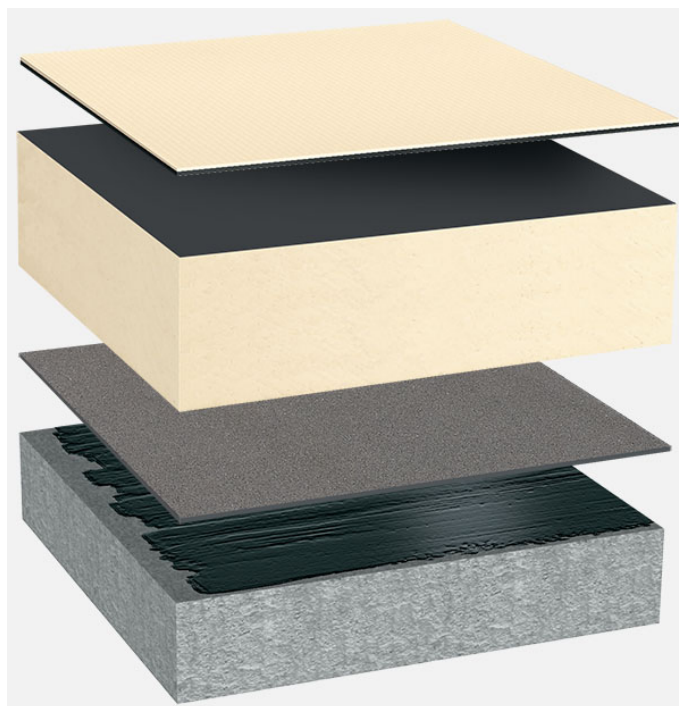
Systemowy układ warstw: BG_PIR-FA_T_01
