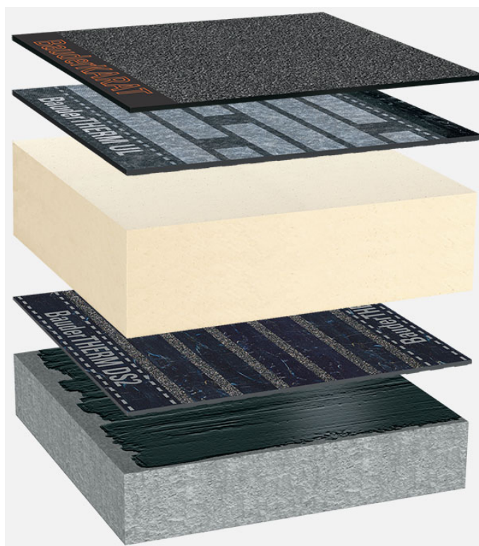
Systemowy układ warstw: BG_PIR-MF_K_01
