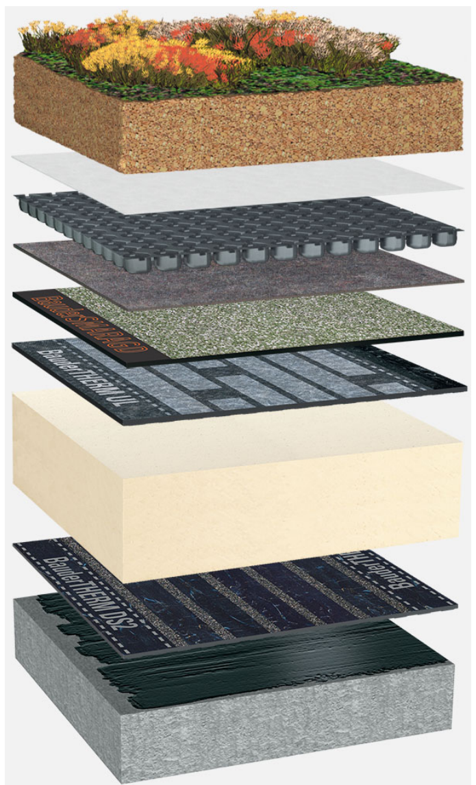
Systemowy układ warstw: BG_PIR-MF_S_01_G125
