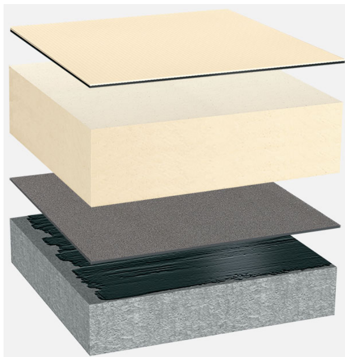
Systemowy układ warstw: BG_PIR-MF_T_01
