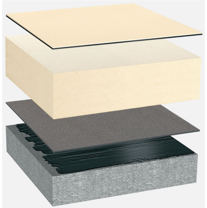
Systemowy układ warstw: BG_PIR-MF_T_01
