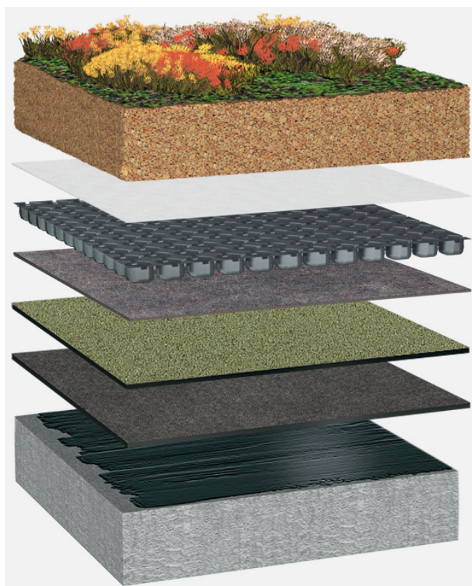
Systemowy układ warstw: BG_P_01_G125
