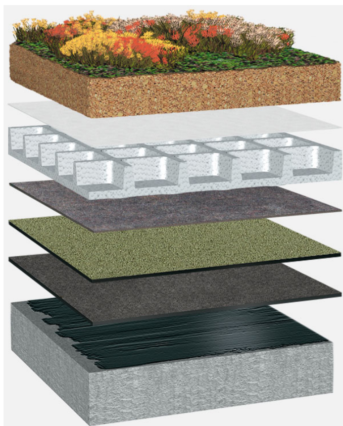
Systemowy układ warstw: BG_P_01_G75
