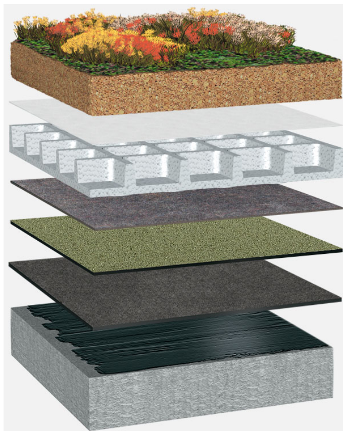
Systemowy układ warstw: BG_P_03_G75
