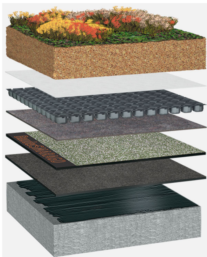
Systemowy układ warstw: BG_S_01_G125
