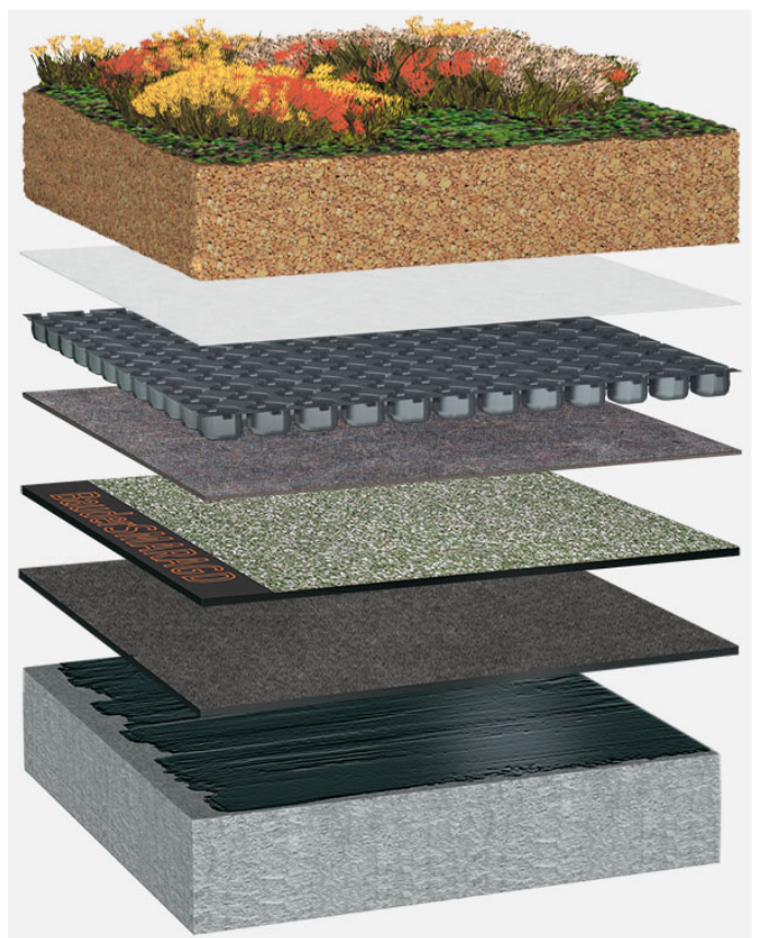
Systemowy układ warstw: BG_S_03_G125
