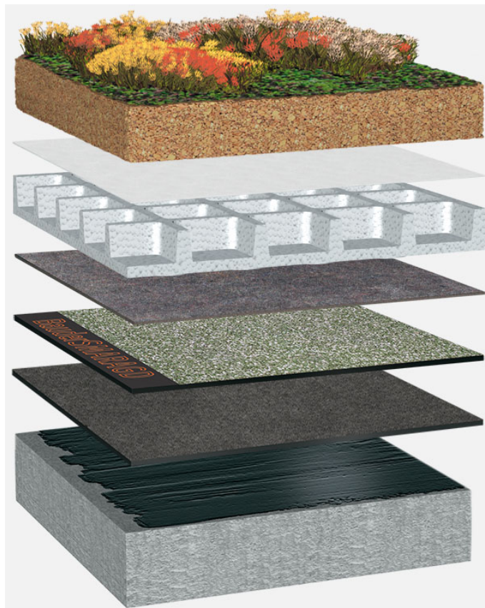
Systemowy układ warstw: BG_S_03_G75
