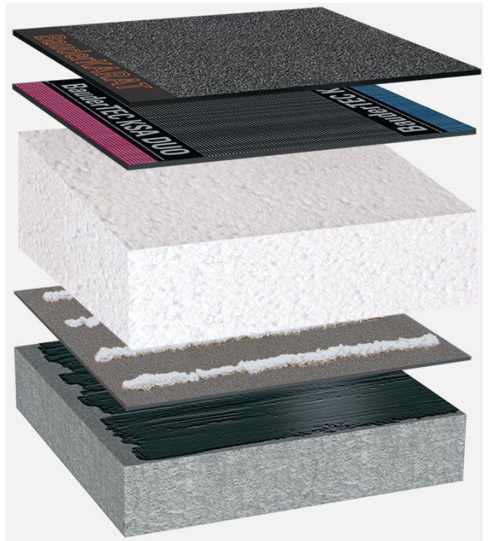
Systemowy układ warstw: BP_EPS-G_K_01
