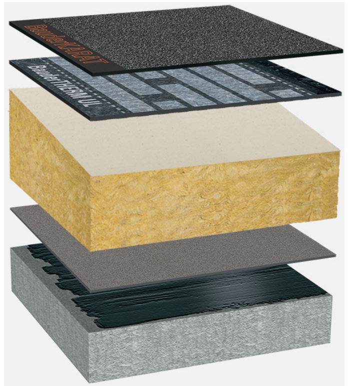
Systemowy układ warstw: BP_MIFA-G_K_01
