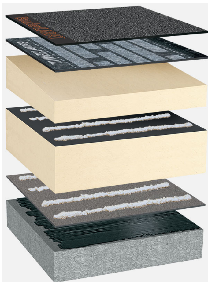
Systemowy układ warstw: BP_PIR-FA_PIR-TG_K_01
