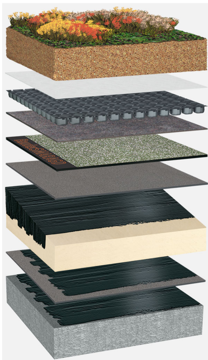
Systemowy układ warstw: BP_PIR-KG_S_01_G125
