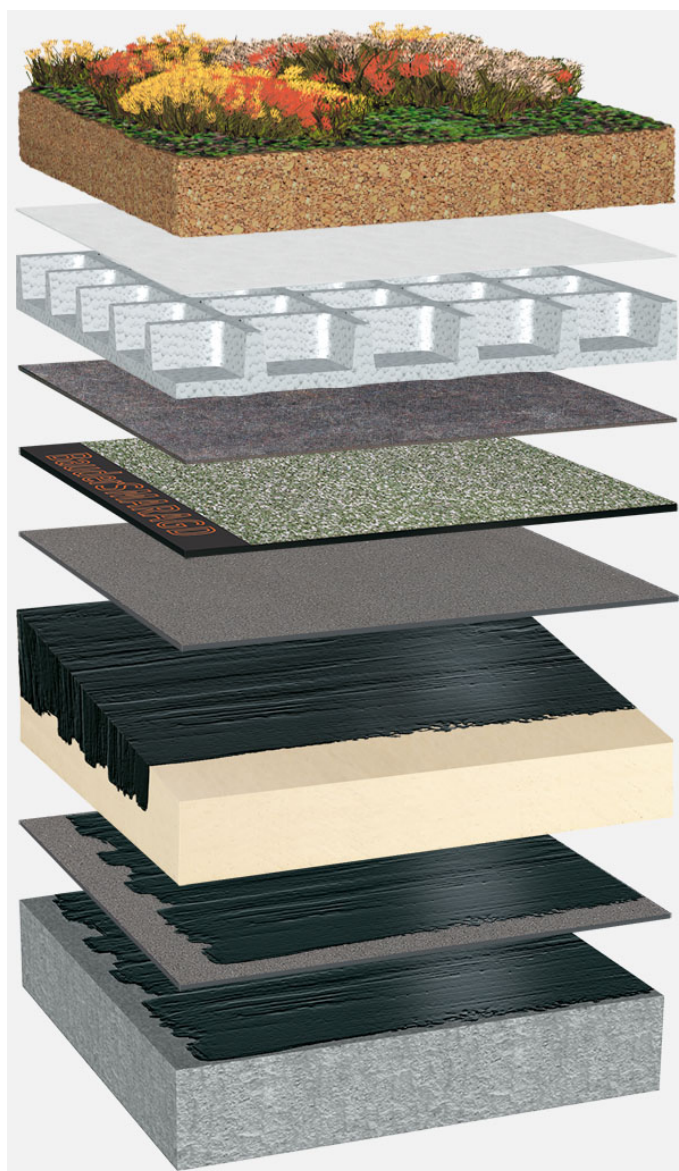
Systemowy układ warstw: BP_PIR-KG_S_01_G75
