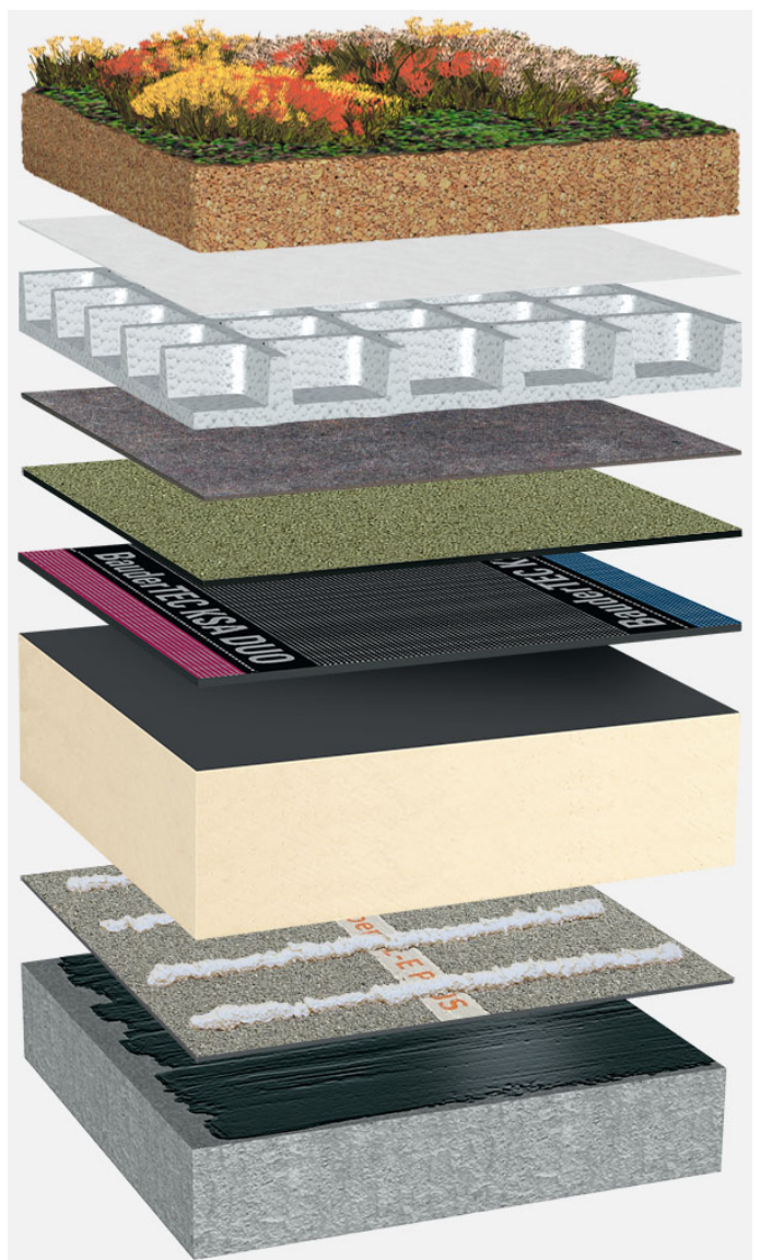
Systemowy układ warstw: BG_PIR-FA_P_01_G75
