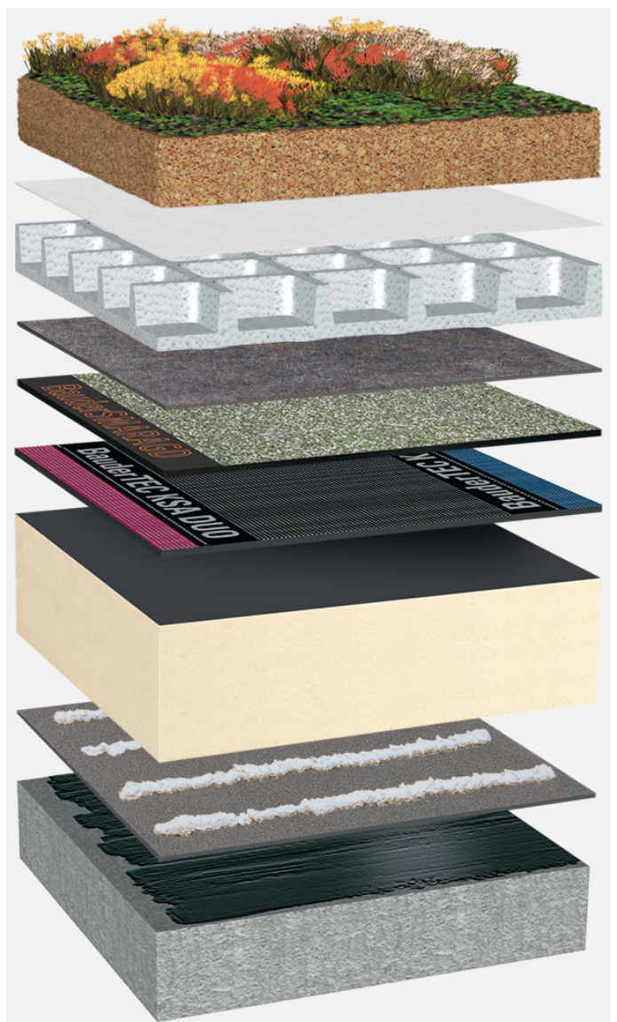
Systemowy układ warstw: BG_PIR-FA_S_01_G75
