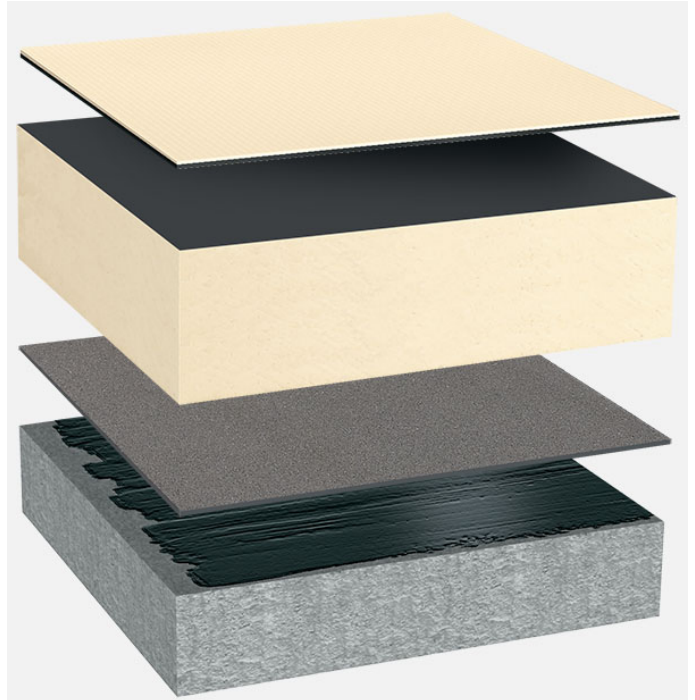
Systemowy układ warstw: BG_PIR-FA_T_01
