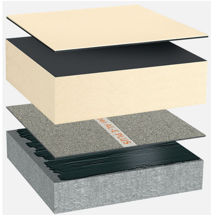
Systemowy układ warstw: BG_PIR-FA_T_02
