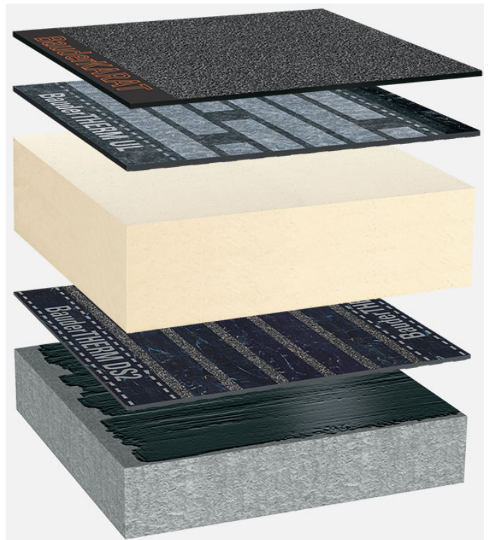
Systemowy układ warstw: BG_PIR-MF_K_01
