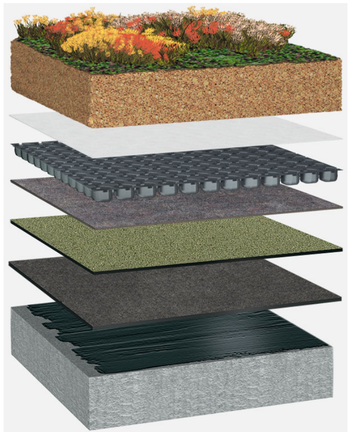
Systemowy układ warstw: BG_P_03_G125
