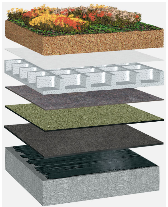
Systemowy układ warstw: BG_P_03_G75
