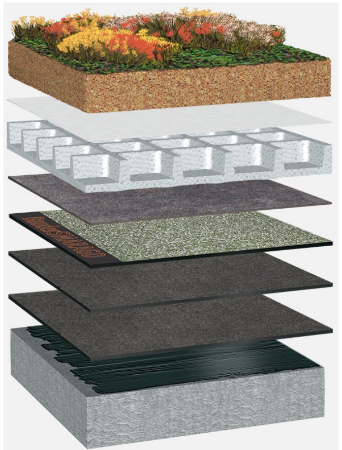
Systemowy układ warstw: BG_S_02_G75
