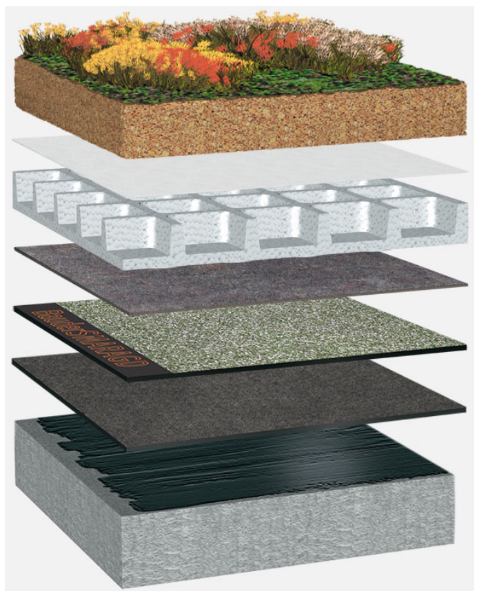
Systemowy układ warstw: BG_S_03_G75
