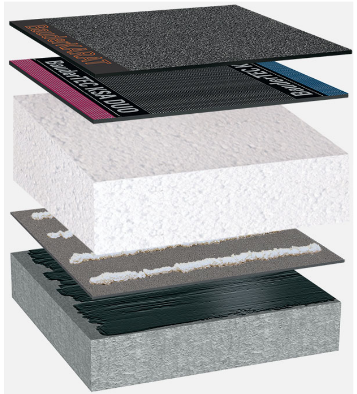
Systemowy układ warstw: BP_EPS-G_K_01
