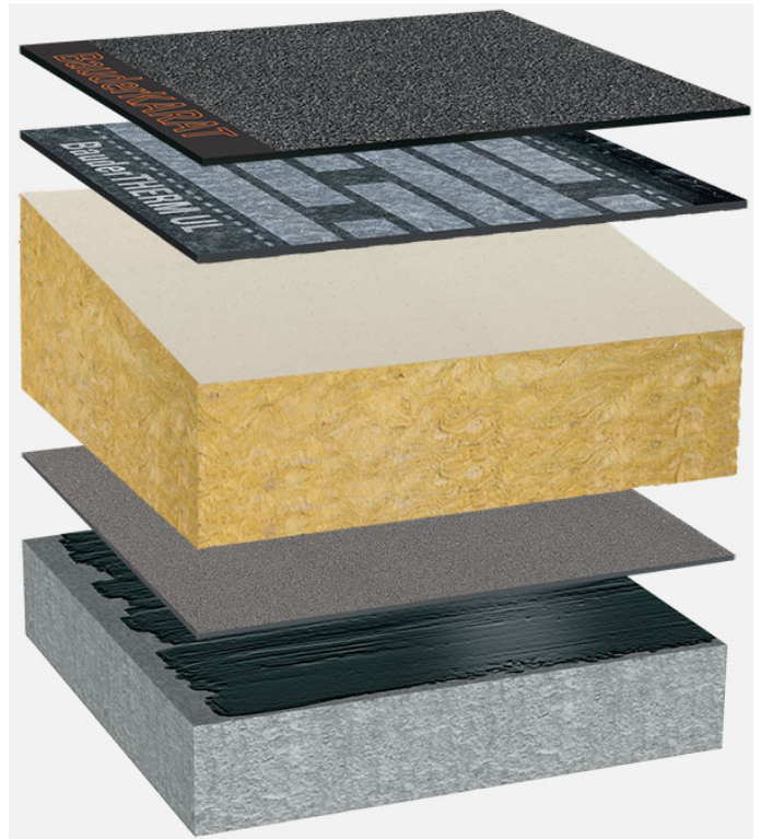
Systemowy układ warstw: BP_MIFA-G_K_01
