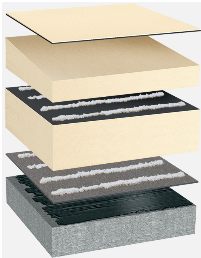
Systemowy układ warstw: BP_PIR-FA_PIR-TG_T_01
