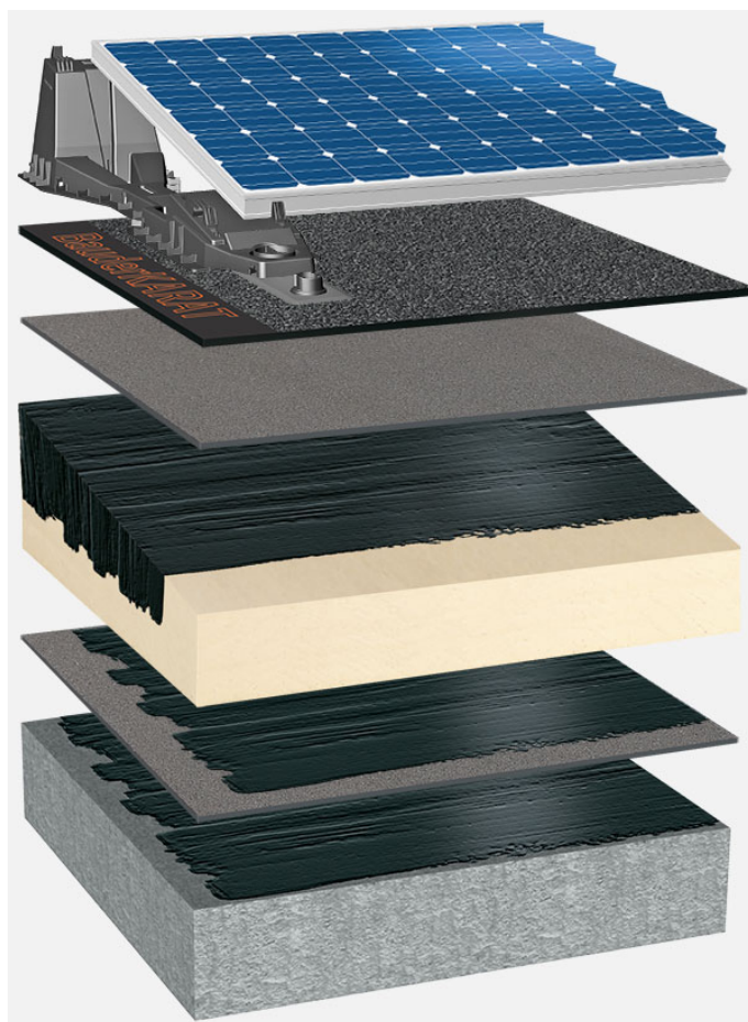
Systemowy układ warstw: BP_PIR-KG_K_01_PVFD
