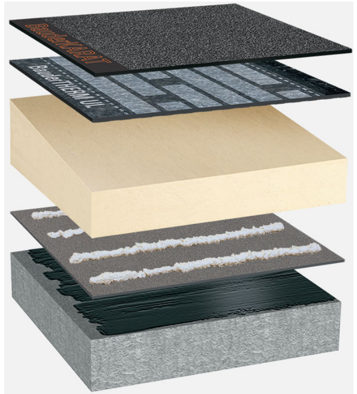
Systemowy układ warstw: BP_PIR-TG_K_01
