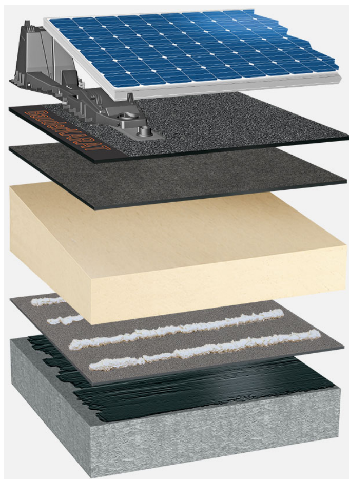
Systemowy układ warstw: BP_PIR-TG_K_01_PVFD
