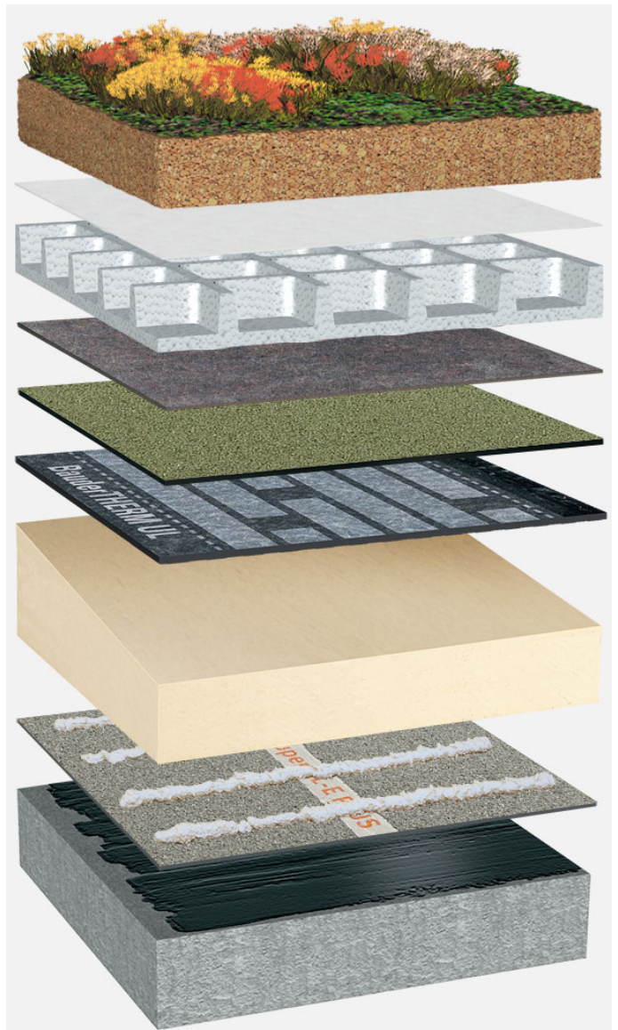
Systemowy układ warstw: BP_PIR-TG_P_01_G75
