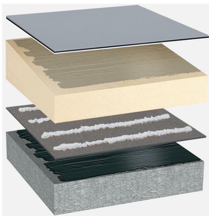
Systemowy układ warstw: BP_PIR-TG_SK_01
