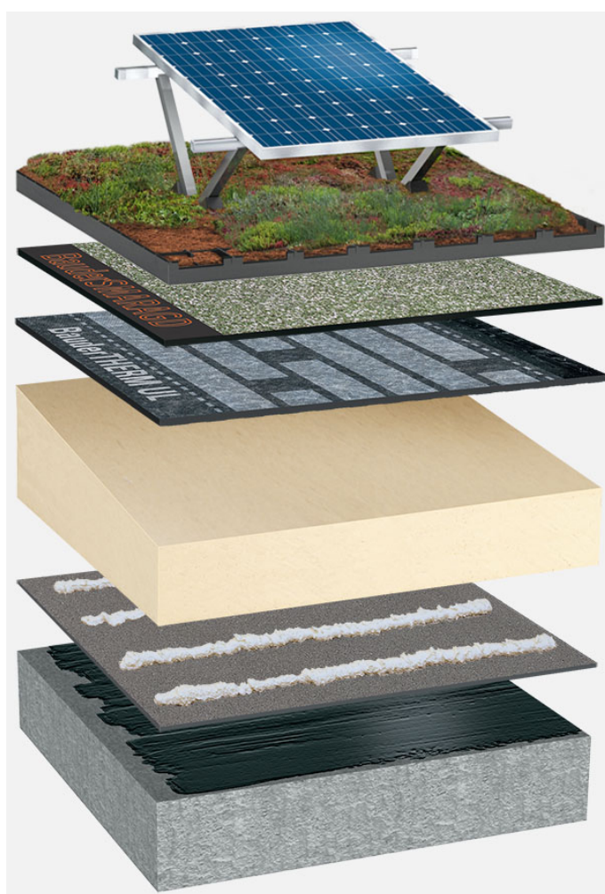
Systemowy układ warstw: BP_PIR-TG_S_01_PVGD
