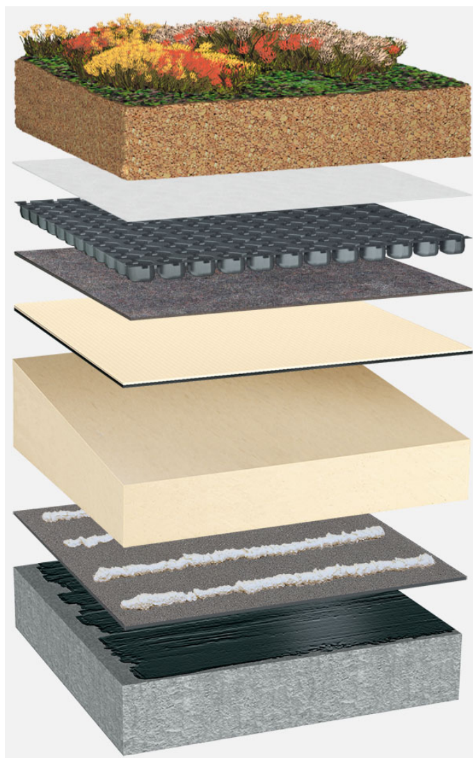
Systemowy układ warstw: BP_PIR-TG_T_01_G125
