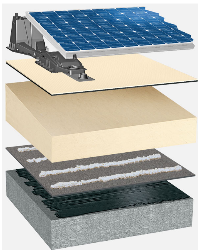
Systemowy układ warstw: BP_PIR-TG_T_01_PVFD
