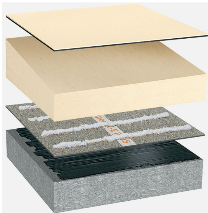
Systemowy układ warstw: BP_PIR-TG_T_02
