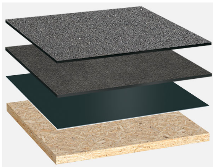
Systemowy układ warstw: HG_B_01
