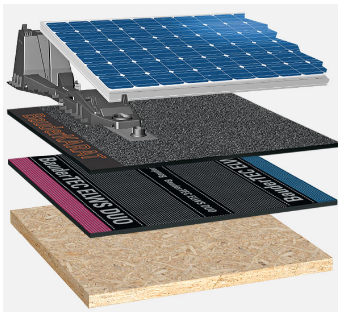
Systemowy układ warstw: HG_K_01_PVFD
