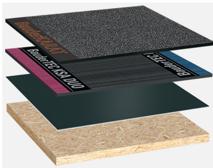
Systemowy układ warstw: HG_K_02
