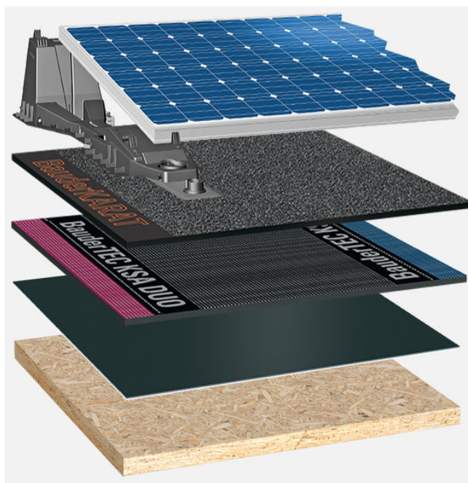
Systemowy układ warstw: HG_K_02_PVFD
