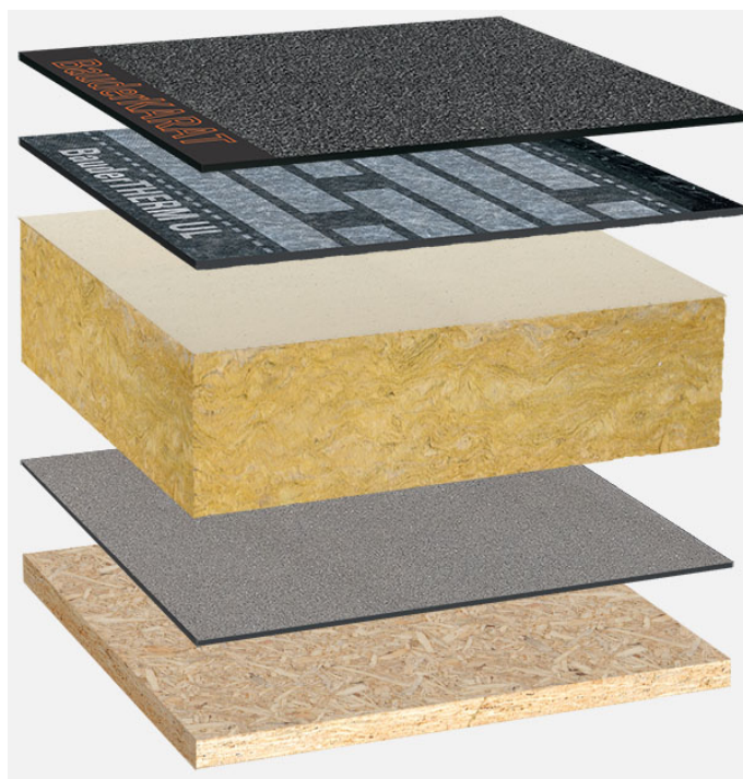
Systemowy układ warstw: HG_MIFA-P_K_01
