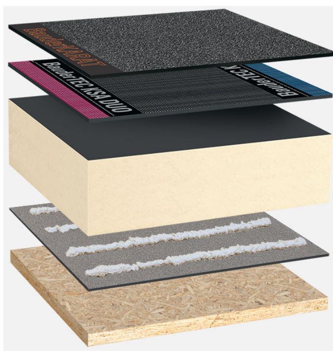
Systemowy układ warstw: HG_PIR-FA_K_01
